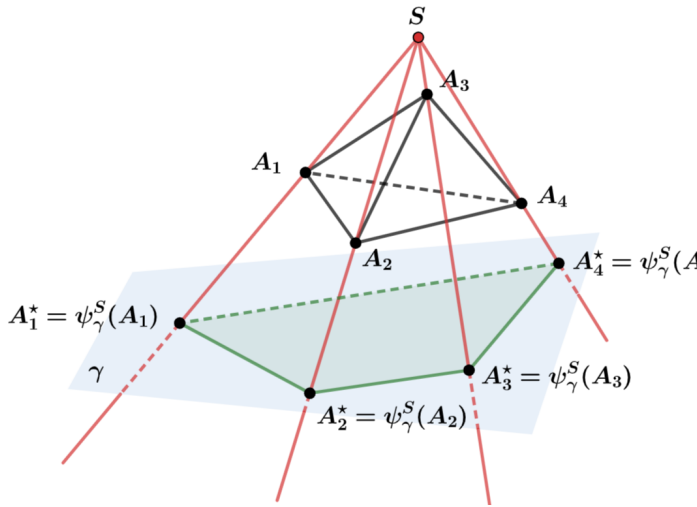
Централно проектиране с краен проекционен център
