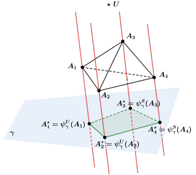
Централно проектиране с безкраен проекционен център
